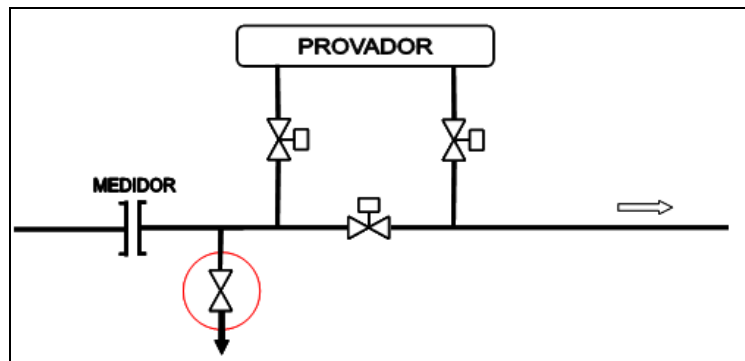
Figura 29 - Válvula de segurança instalada em posição não conforme ao API
