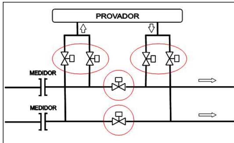
Figura 24 - Válvulas intermediárias e válvulas de entrada e saída do provedor - provedor conectado a mais de uma linha de medição
