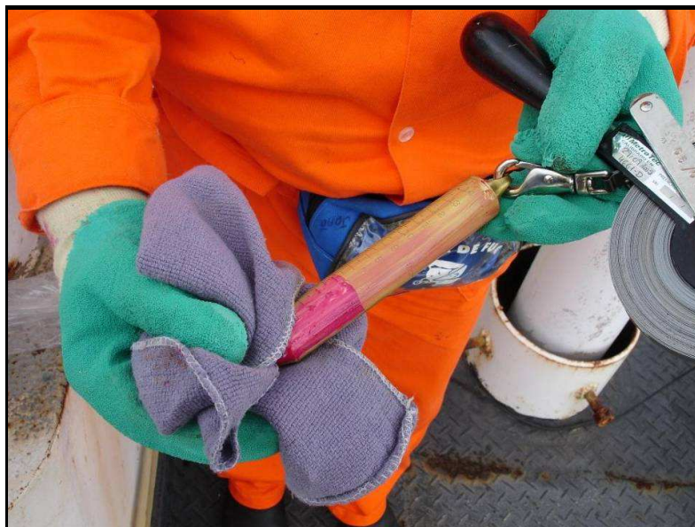
Figura 9 - Prumo da trena com pasta d'água
