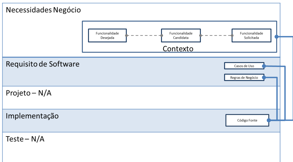
Figura 18 – Arquitetura de rastreabilidade para o processo instanciado.
