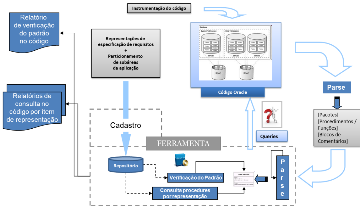
Figura 20 – Visão mais detalhada da ferramenta
