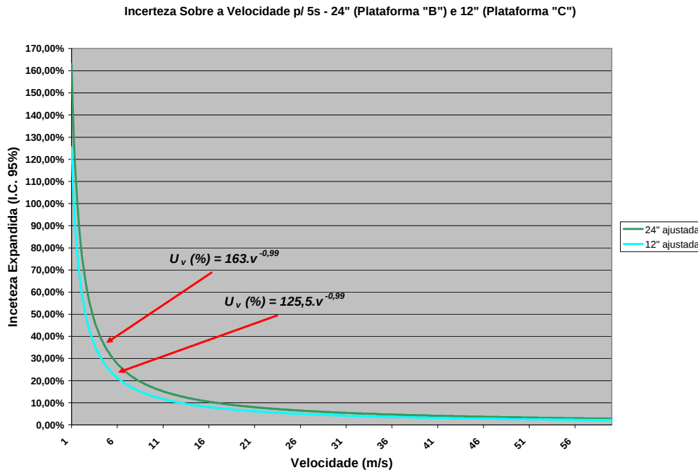
Figura 14 - Incerteza expandida da velocidade do escoamento para 5 s (I.C. \approx 95 %): medidores de 12\" e 24\" (Elaboração Própria)
