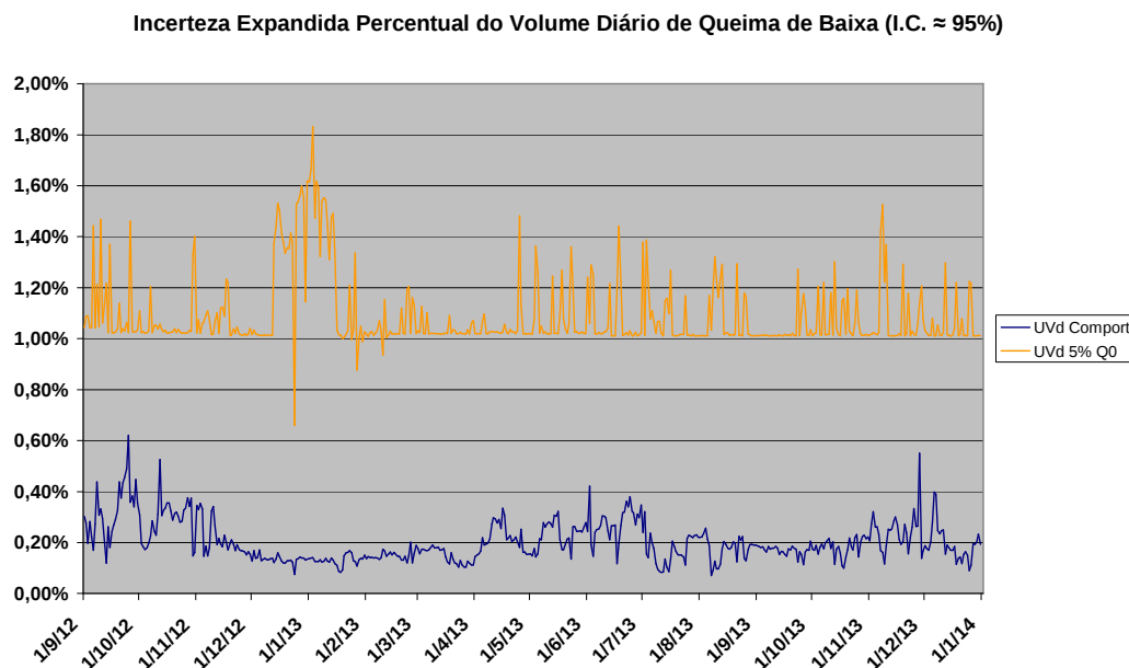
Figura 18 - Comparação entre as incertezas dos volumes queimados de baixa pressão (Elaboração Própria)
