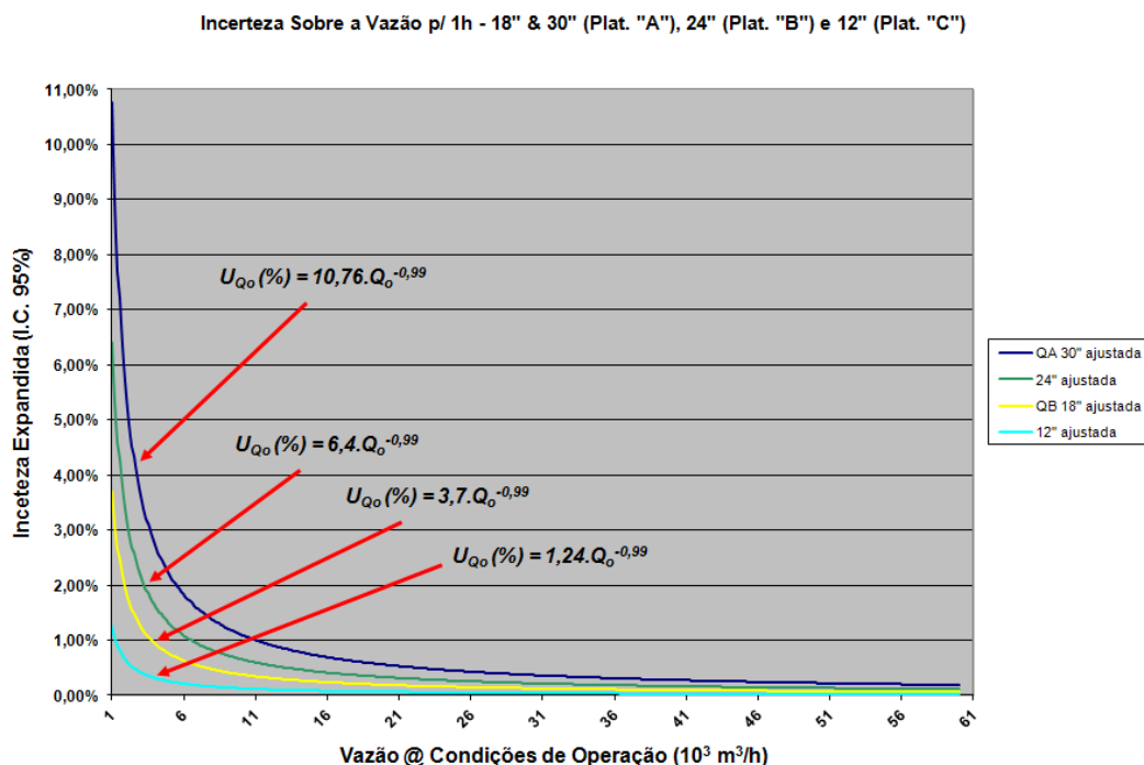
Figura 15 - Incerteza da vazão volumétrica não-corrigida para 1 h – medidores de 12”, 18”, 24” e 30” (Elaboração Própria)
