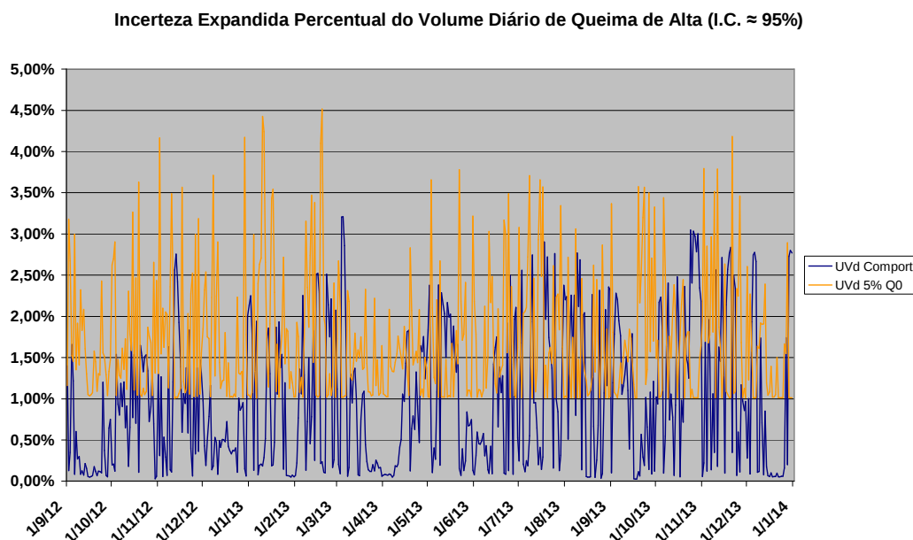
Figura 17 - Comparação entre as incertezas dos volumes queimados de alta pressão (Elaboração Própria)
