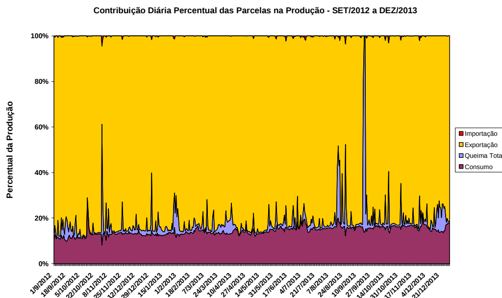
Figura 20 - Contribuição diária das correntes de produção em 16 meses – Plataforma “A”
