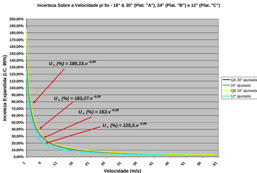
Figura 16 - Incerteza da velocidade do escoamento para 5 s, medidores de 12", 18", 24" e 30" (Elaboração Própria)
