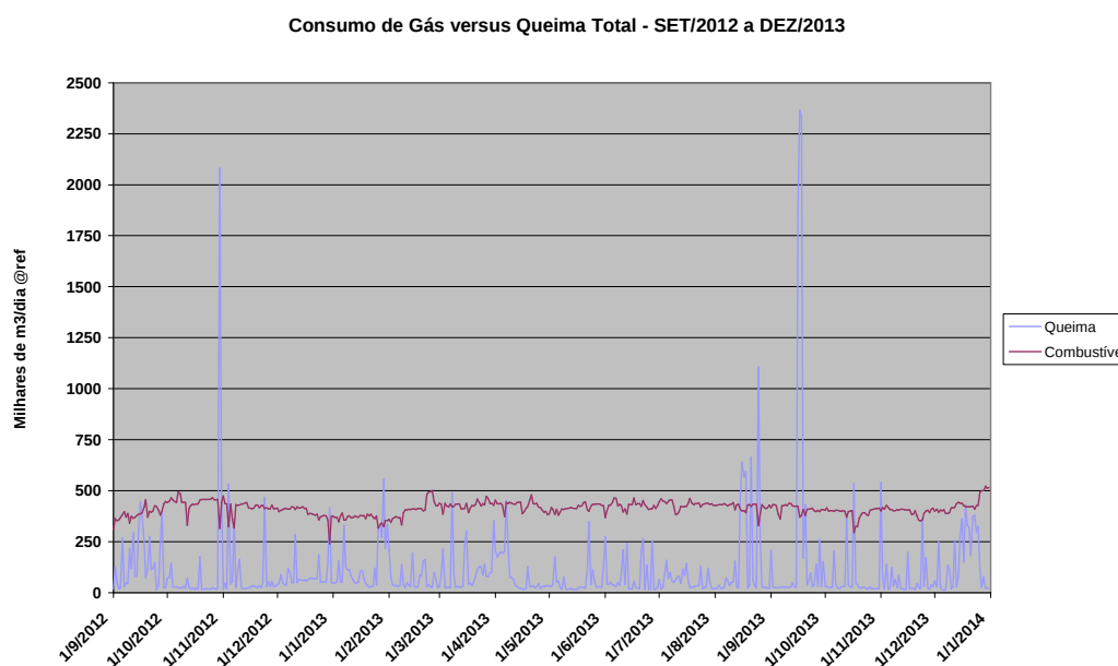
Figura 19 - Comparação entre volumes queimados e consumidos em 16 meses – Plataforma “A”
