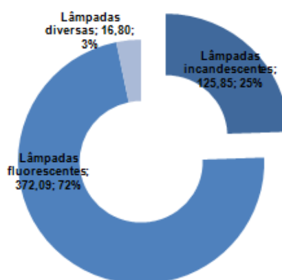
Figura 5.6 - Tipos de lâmpadas e seu consumo de energia total
