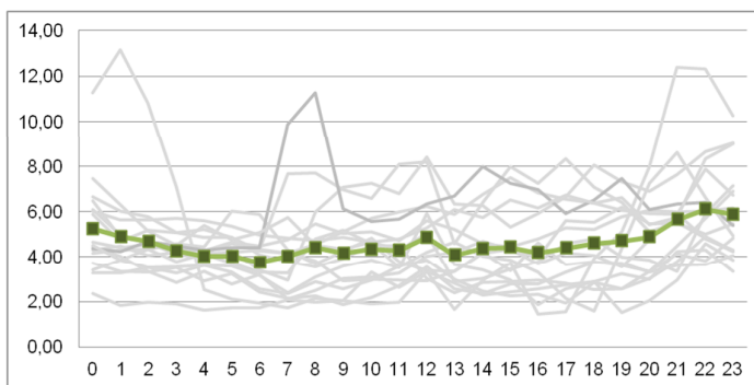
Figura 5.12 - Curva média mensal de carga (kWhxh) dos consumidores beneficiados da adesão à tarifa branca (faixa: 0-150 kWh)
