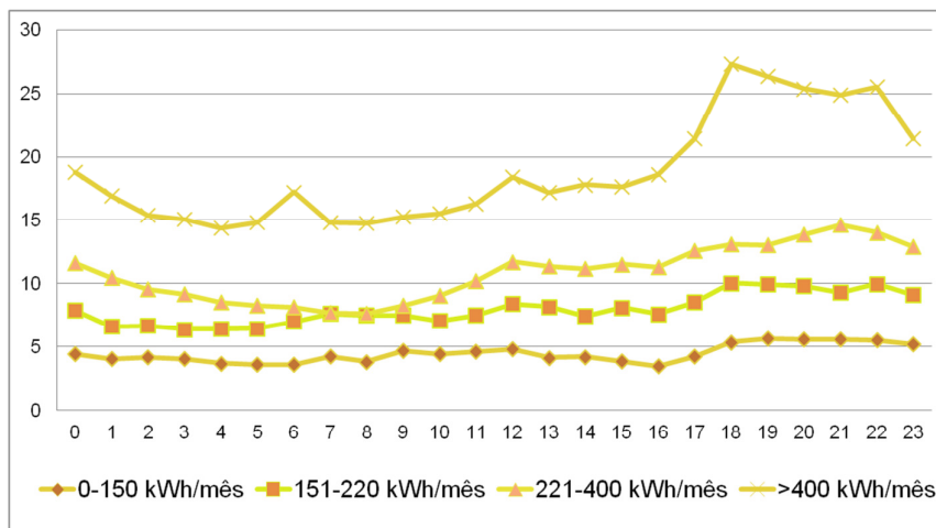
Figura 5.61 - Perfil médio dos consumidores com potencial de se beneficiar com a adoção da tarifa branca por faixa de consumo
