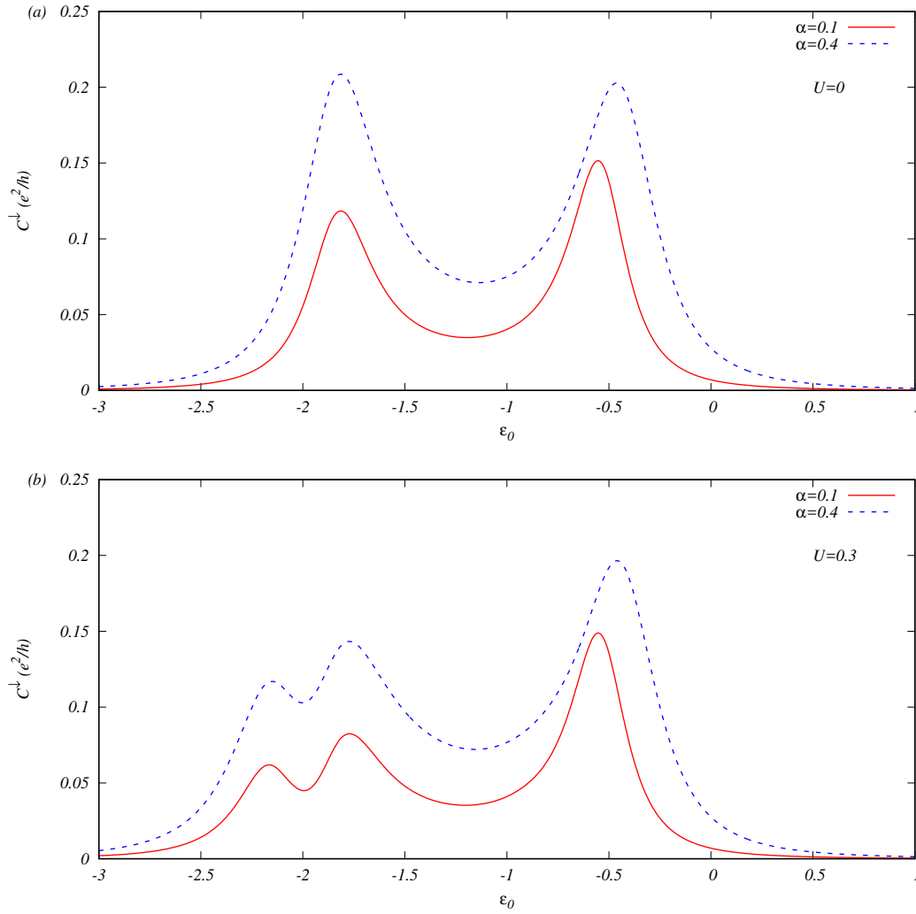
Figura 4.9: Condutância spin para baixo, C^\downarrow , no contato i = 1 como função do potencial de porta, \epsilon_0 para dois valores de \alpha . Painel (a) com repulsão Coulombiana U = 0 e painel (b) com U = 0.3 .
