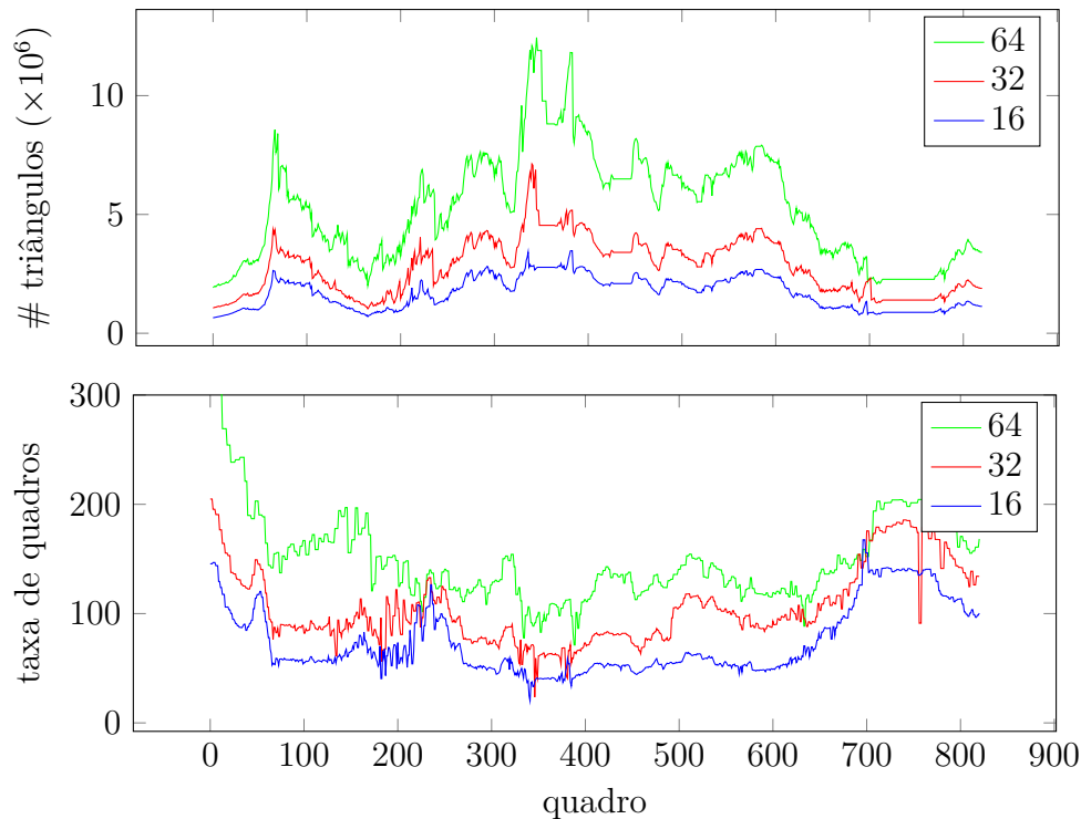
Figura 5.3 – Influência do tamanho do patch no número de triângulos gerados e na performance ao longo do caminho: patches maiores aumentam o número de triângulos gerados, porém entregam um melhor desempenho. A memória de GPU usada é a mesma.
