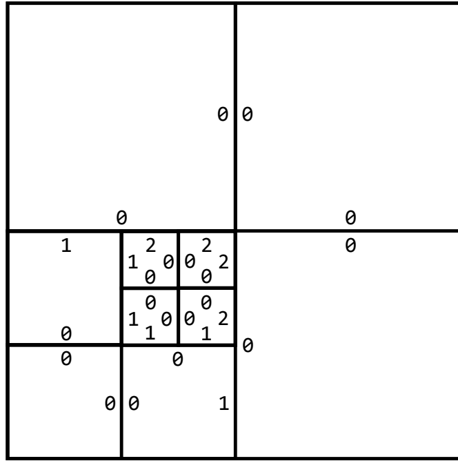
Figura 3.4 – Diferença de níveis ao longo da borda do ladrilho. Para cada ladrilho selecionado, os ladrilho vizinhos são checados; se o vizinho for do mesmo nível ou maior, a diferença é zero. Caso o ladrilho vizinho seja de um nível menor, a diferença é computada.
