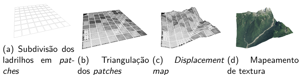
Figura 3.7 – Pipeline de GPU da nossa proposta: A CPU seleciona e envia os ladrilhos para a GPU. Para cada patch , os níveis de triangulação são selecionados; cada vértice gerado recebe a sua altura respectiva, e a textura é mapeada sobre os triângulos gerados.
