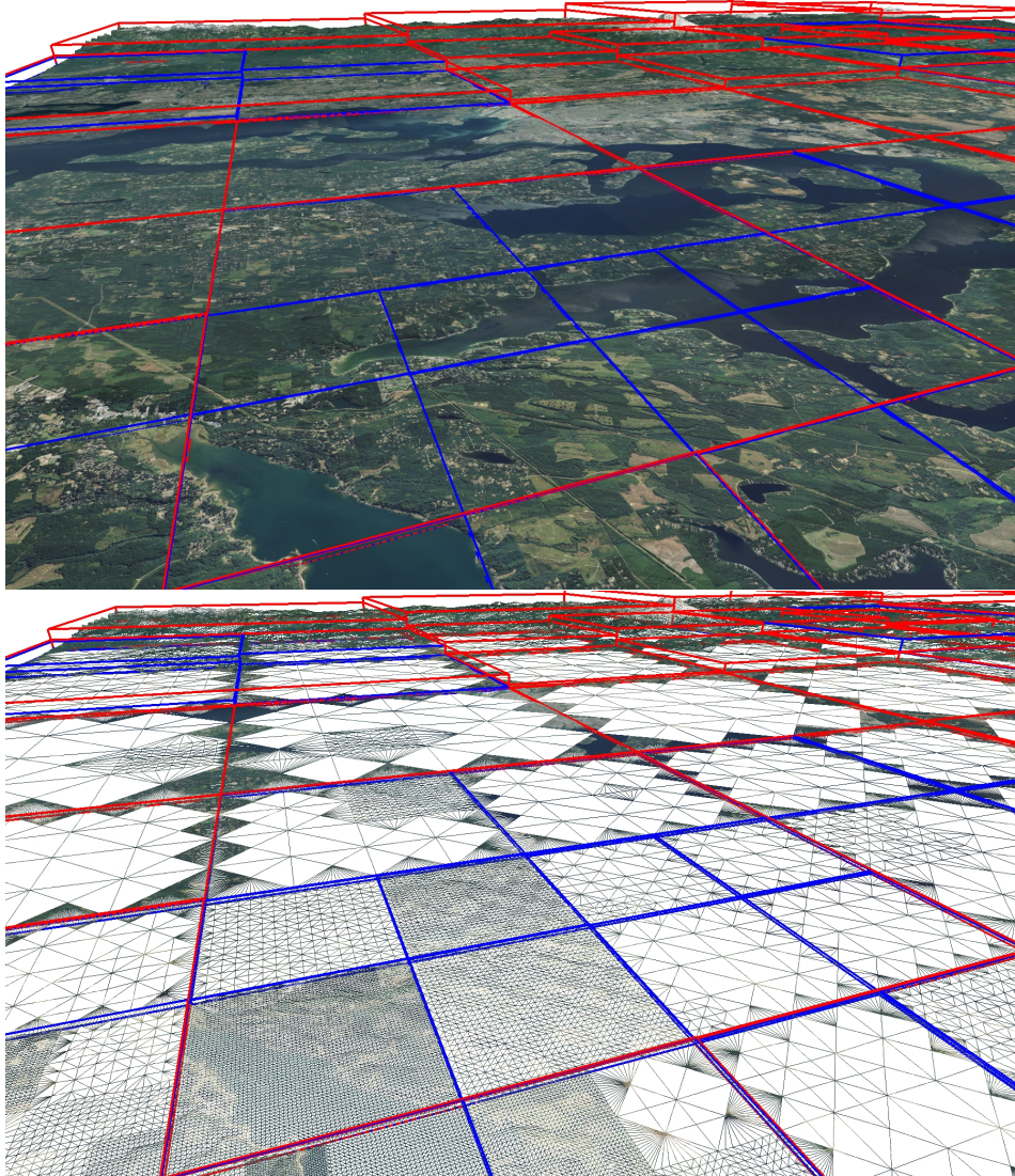
Figura 3.6 – Correspondência 1-para- n : um ladrilho de geometria para múltiplos de textura. Um ladrilho virtual de geometria é desenhado para cada ladrilho de textura; todos os ladrilho virtuais compartilham o mesmo dado de elevação.
