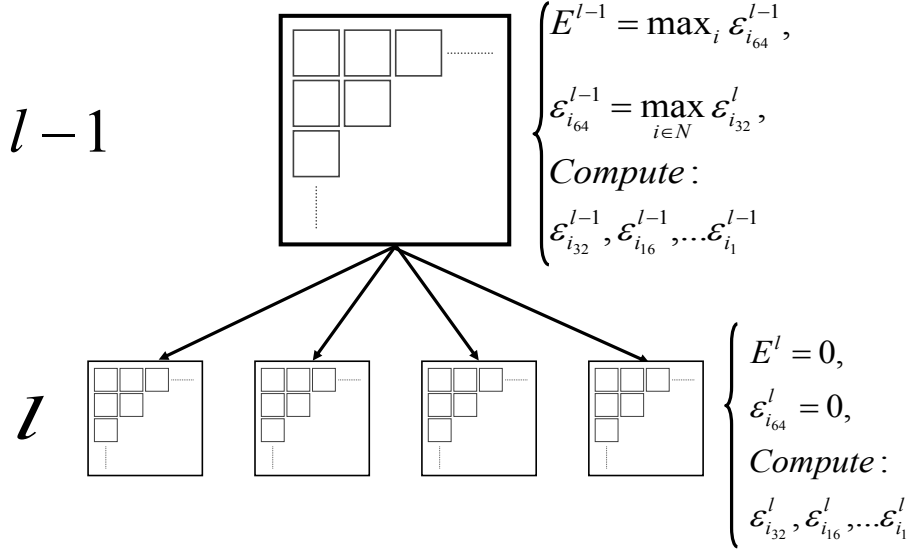
Figura 3.3 – Cálculo do erro no espaço do objeto: nos nós folha, o erro de cada patch na triangulação máxima é zero. Os erros dos patches nos níveis superiores são herdados dos níveis inferiores. O erro associado a cada ladrilho é o erro máximo dos seus patches na triangulação máxima.
