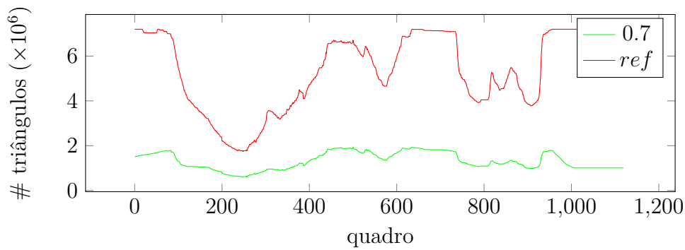
Figura 5.6 – Comparação entre os triângulos gerados pela malha completa( ref ) e os gerados pelo algoritmo de LOD com uma tolerância de 0.7 pixels.
