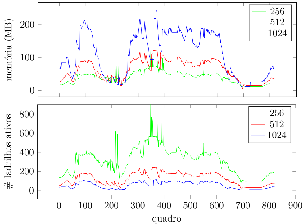
Figura 5.2 – A influência do tamanho do ladrilho na quantidade de memória de GPU necessária: ladrilhos pequenos demandam menos memória, porém aumentam a quantidade de trabalho em CPU.
