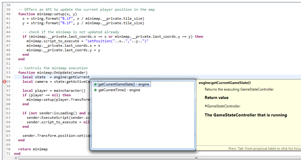
Figura 5.15 – Editor de código exibindo as funcionalidades de Syntax Coloring e Code Assistance .
