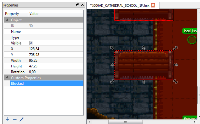
Figura 5.22 – Através da propriedade Blocked é possível marcar objetos como barreiras físicas para o jogador.
