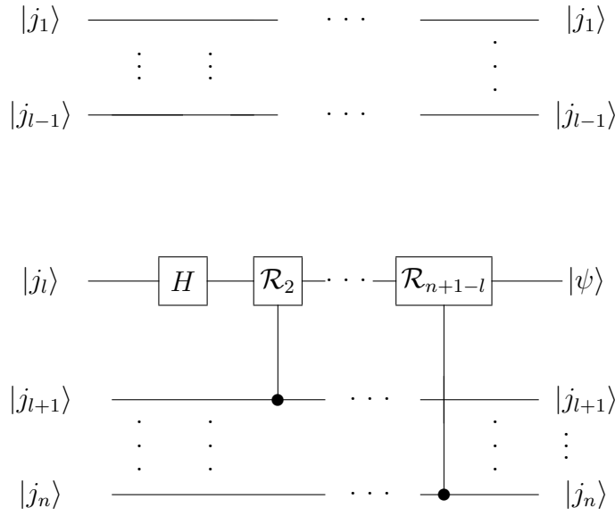
Figura 7.2: Circuito com portas \mathcal{R} e de Hadamard
