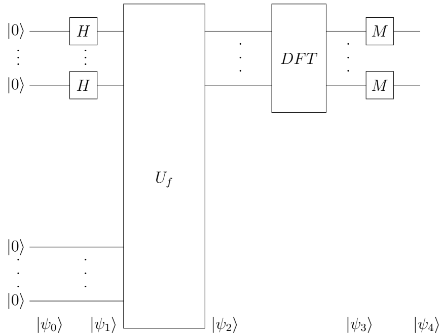
Figura 7.1: Circuito básico da parte quântica
