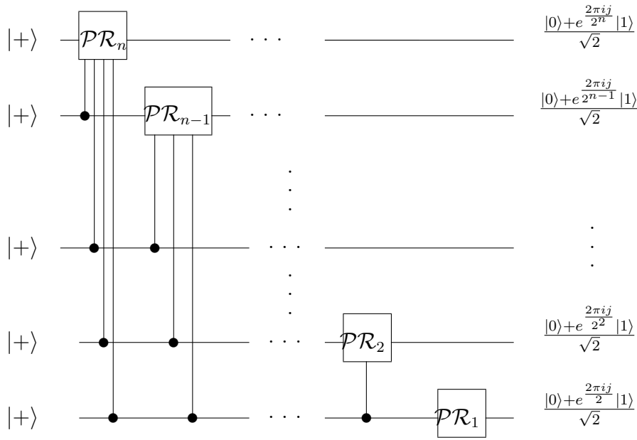
Figura 7.3: Circuito com portas \mathcal{PR} e de Hadamard
