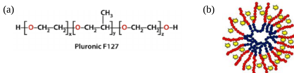
Figura 1.6. (a) Estrutura química Pluronic F-127, x \approx z \approx 100 , y \approx 65 ; (b) micelas de Pluronic. Moléculas de água em amarelo. Figura modificada de (Vilsinska, 2014)
