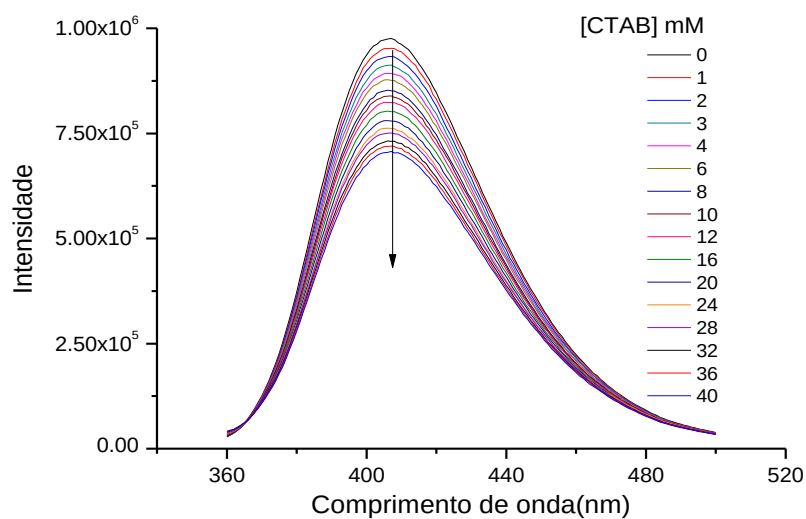
Figura 4.8. Espectros de fluorescência da solução de NFX 8 \mu M titulada com concentrações crescentes de CTAB (tampão fosfato de 10 mM, pH 7,4)
