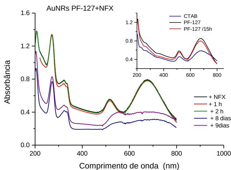
Figura 4.24. Espectros de absorção referentes ao nano bastões estabilizados com Pluronic F-127 0,2 mM, antes e após adição de NFX 20 µM.
