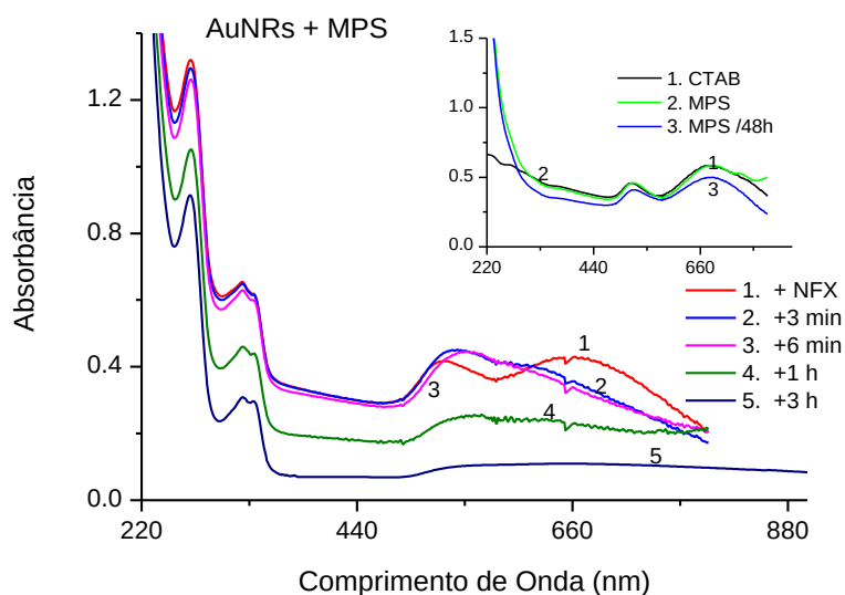
Figura 4.22. Espectros de absorção/extinção referentes aos AuNRs estabilizados com MPS, antes e após adição de NFX 20 \mu\text{M} .
