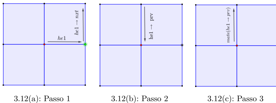
Figura 3.12: Algoritmo de adjacência
