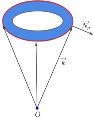
Figura 4.1: Curva silhueta
