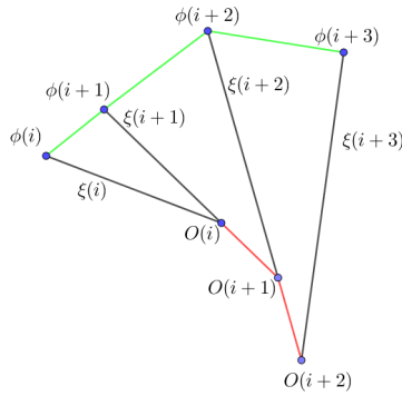
Figura 4.8: Polígono observador.
