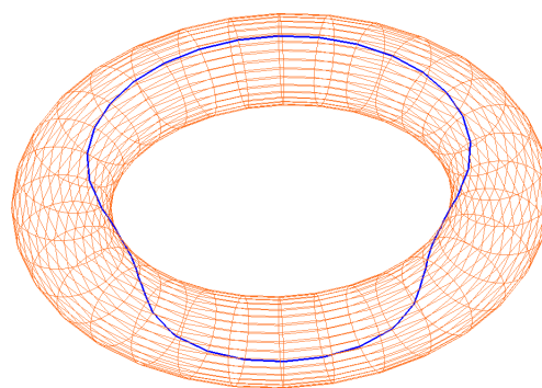
4.10(b): Silhueta não planar
