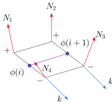
Figura 4.9: Silhueta.
