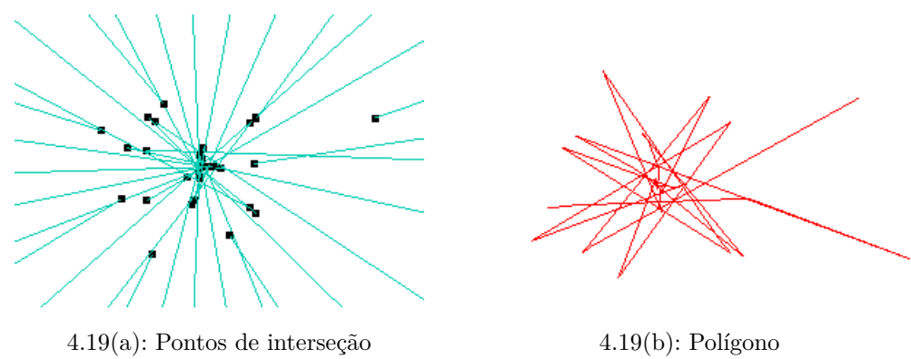
Figura 4.19: Polígono observador na malha circular - toro
