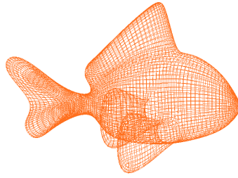
Figura 4.21: Malha Peixe
