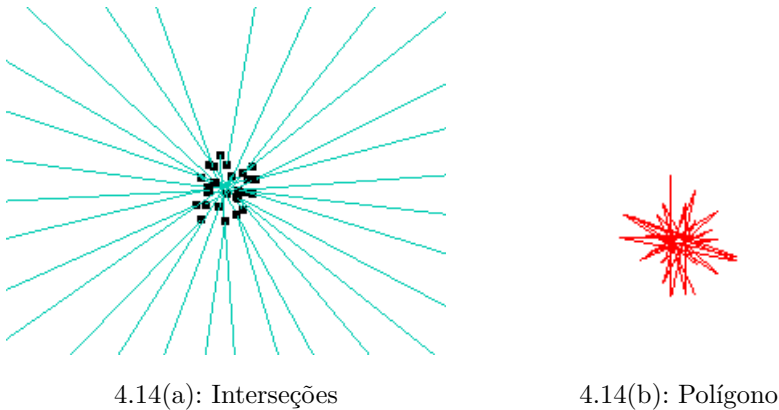
Figura 4.14: Polígono malha circular - hiperbolóide
