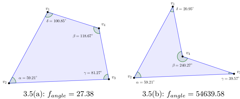
Figura 3.5: f_{angle} na face
