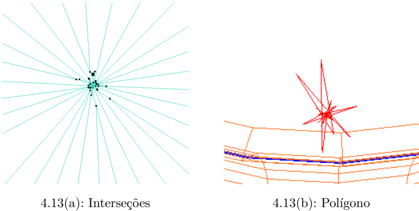
Figura 4.13: Polígono malha cônica - hiperbolóide
