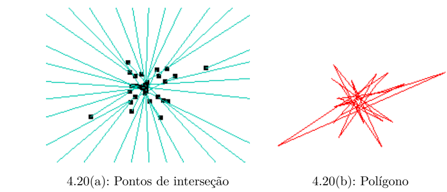
Figura 4.20: Polígono observador na malha cônica - toro
