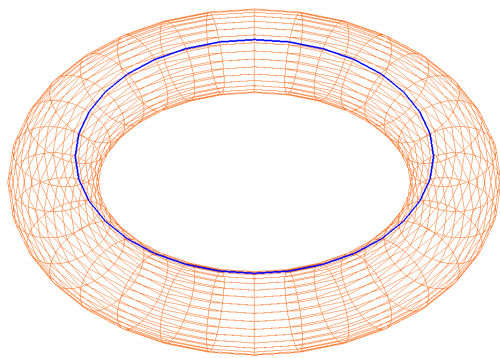
4.10(a): Silhueta planar
