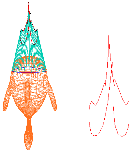
4.22(a): Pontos de in- 4.22(b): Polígono observador terseção
