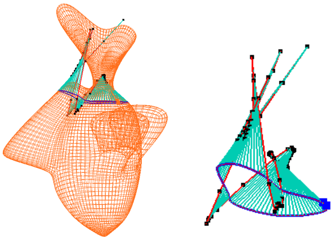
4.23(a): Pontos de interseção 4.23(b): Polígono
