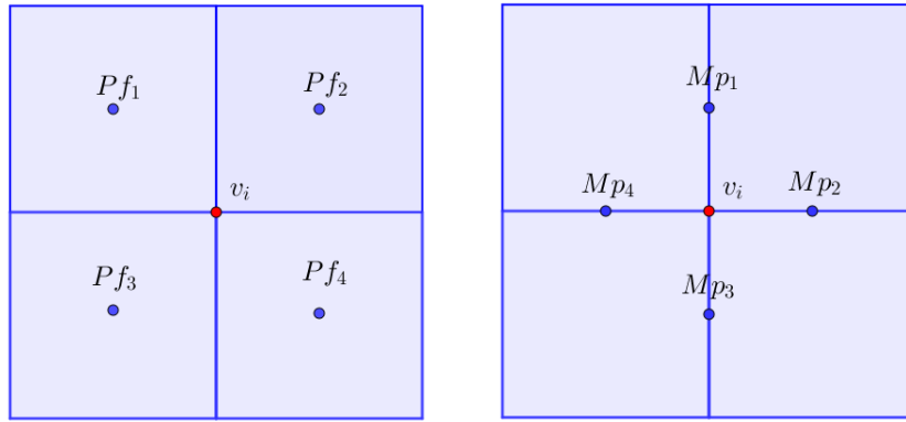
2.5(a): Média dos pontos face F
