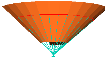
Figura 4.7: Poliedro tangente osculante discreta
