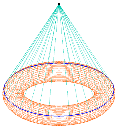
4.18(a): Malha circular
