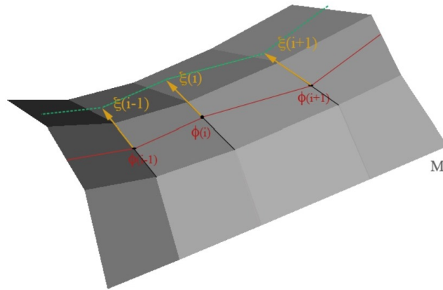
Figura 4.6: Campo de Darboux paralelo [4]
