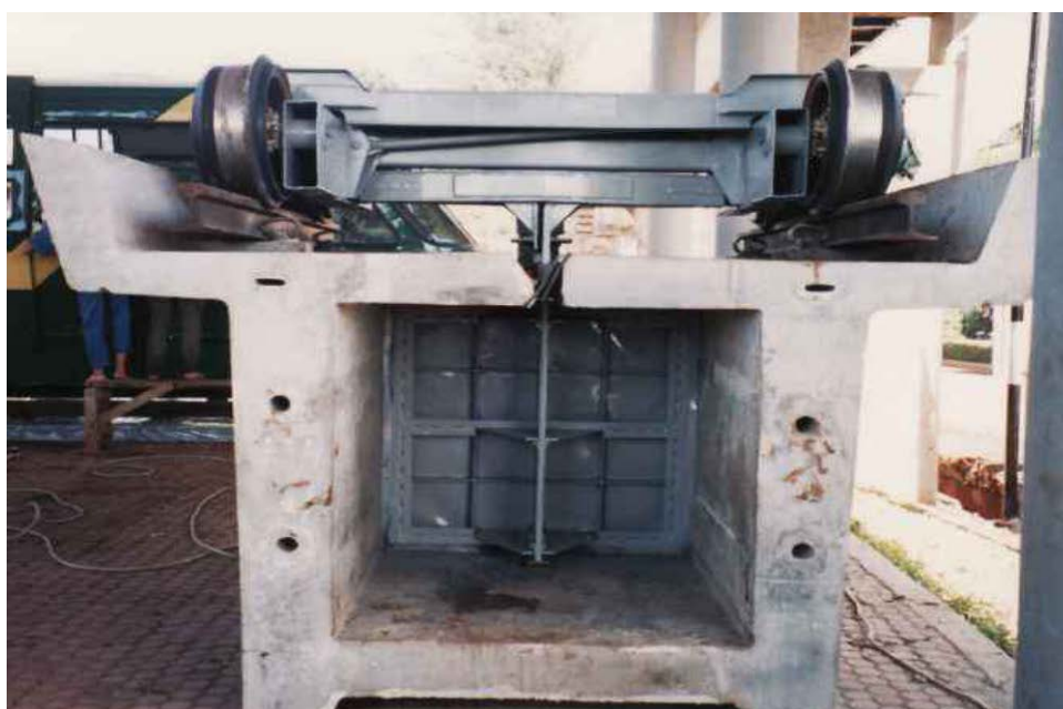
Figura 1 – Detalhe da Vela Invertida no Interior da Viga Pré-Moldada (Coester, 2014).
