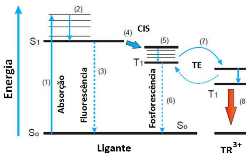
Figura 9- Representação do mecanismo de transferência de energia entre um ligante orgânico e um íon terra-rara [44, 45].
