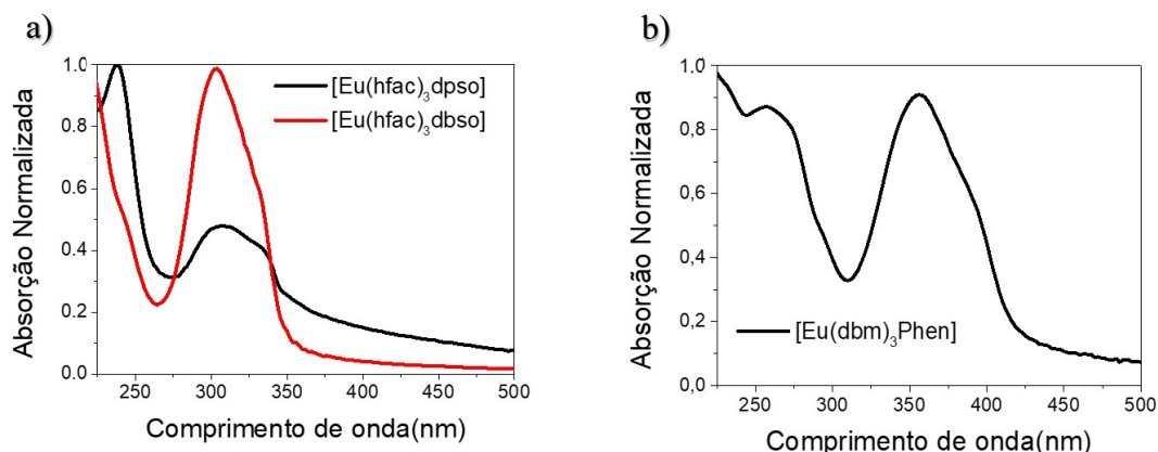
Figura 27- a) Espectros de absorção normalizados dos complexos [\text{Eu}(\text{hfac})_3\text{dpso}] , [\text{Eu}(\text{hfac})_3\text{dbso}] e b) [\text{Eu}(\text{dbm})_3\text{phen}] na forma de filmes finos.
