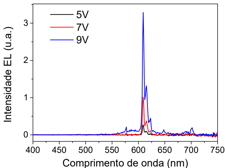
Figura 34- Espectro de EL do OLED de arquitetura 2.
