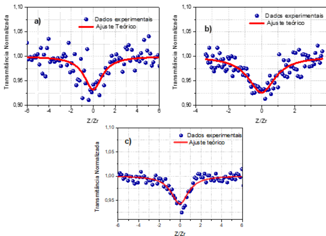
Figura 7.13: Variação da transmitância normalizada para uma amostra de NbS 2 com muitas camadas (+10 layers) através do Z-Scan no experimento de íris aberta, nas intensidades de (a) 50, (b) 80, (c) 120 W/cm². Para esta medida foi utilizado um laser de Nd:YAG, com emissão em 1064nm, mode-locked, com pulsos de 100ps de duração e taxa de repetição de 100MHz. A linha vermelha apresenta ajuste teórico.
