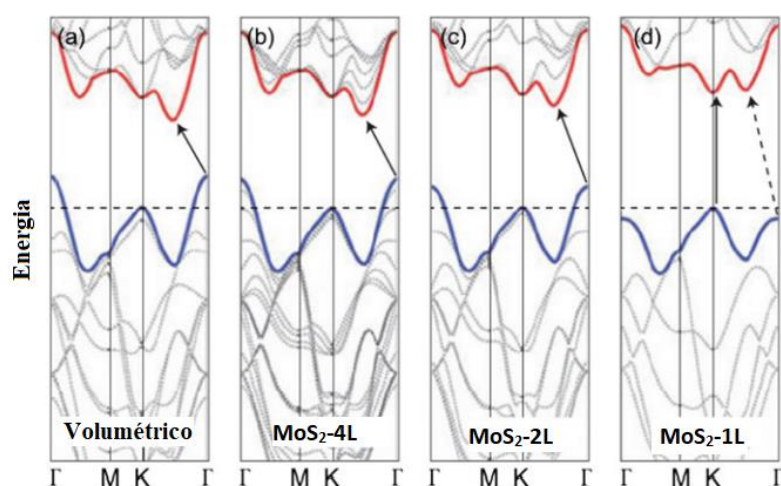
Figura 6.3: Estruturas de banda eletrônica, em função do vetor de onda, do \text{MoS}_2 dependente da quantidade de camadas. As linhas vermelhas e azuis representam a banda de condução e a valência do \text{MoS}_2 , respectivamente. A seta sólida representa as transições de mais baixa energia, para o caso de monocamada a transição é direta (linha vertical). A seta pontilhada indica no caso de monocamada refere-se a uma transição indireta. Adaptado de [70].
