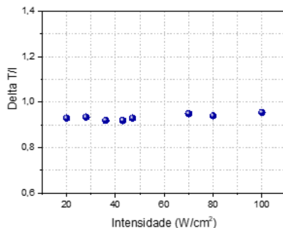
Figura 7.14 Variação do delta T por I função da intensidade I para a amostra NbS 2 +10L no experimento Z-Scan com íris aberta.
