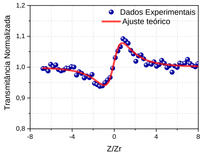
Figura 8.4: Variação da transmitância normalizada para uma amostra do \text{CS}_2 medida através da técnica Z-Scan. A linha vermelha representa o ajuste teórico. Laser da mongagem operando em 94ps; 10Hz
