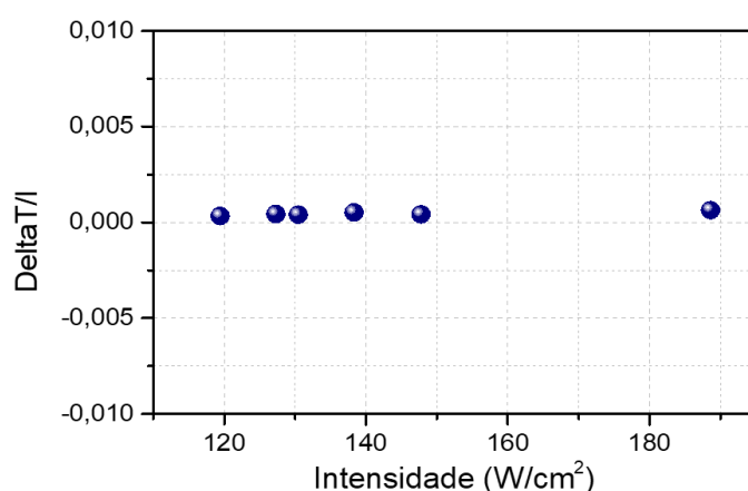
Figura 7.8: Variação do delta T por I em função da intensidade de \text{NbS}_2 monocamada.
