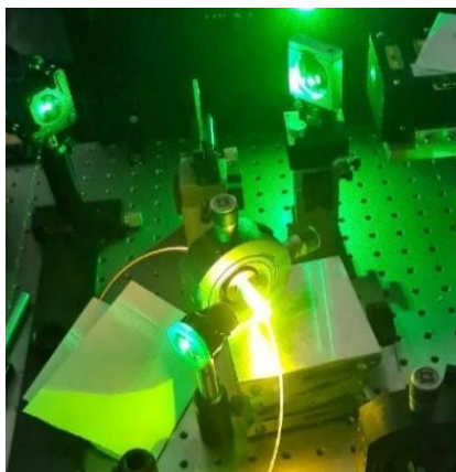
Figura 4.6: Montagem do laser aleatório em suspensão HPC+CNC+Rh6G na configuração de guia onda.
