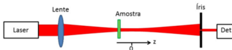
Figura 5.3: Ilustração do esquema experimental da varredura-z (Z-Scan), na qual a amostra se desloca ao longo da direção de propagação do feixe (eixo z ). Adaptado de [40].
