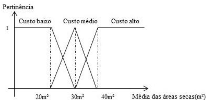
Figura 20: Função de pertinência da variável média das áreas secas.
