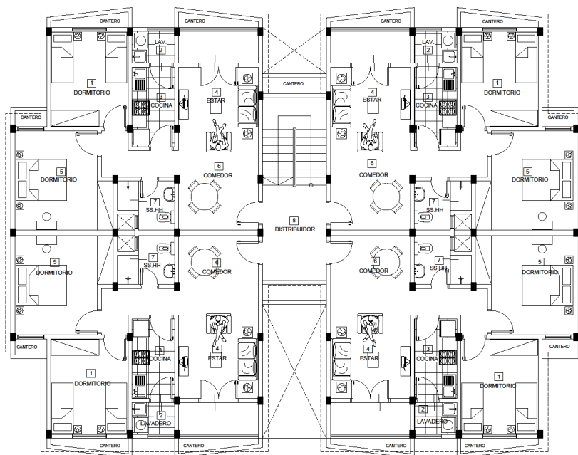
PLANTA TIPO EQUIPADA NÍVEL +2.83 +5.76
