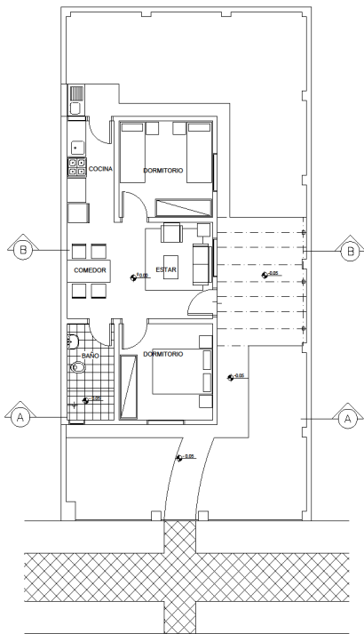
PLANTA EQUIPADA ESC. 1:50 TIPOLOGIA VIVIENDAS 2 DORMITORIOS - Area: 48.00 m2
