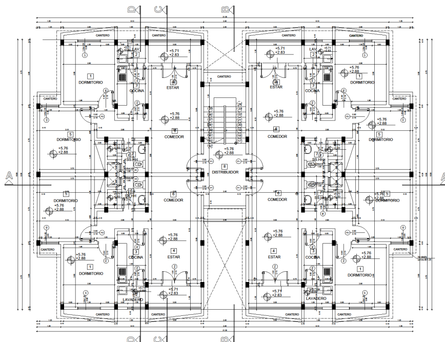
PLANTA TIPO ACOTADA NÍVEL +2.88 +5.76
