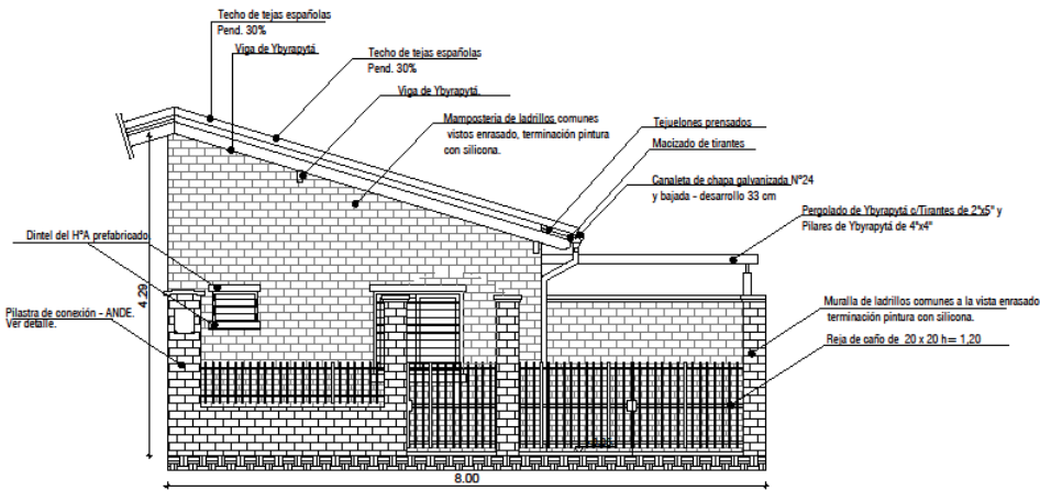
FACHADA FRONTAL. ESC. 1:50 TIPOLOGIA VIVIENDAS 2 DORMITORIOS - Area: 48.00 m2
